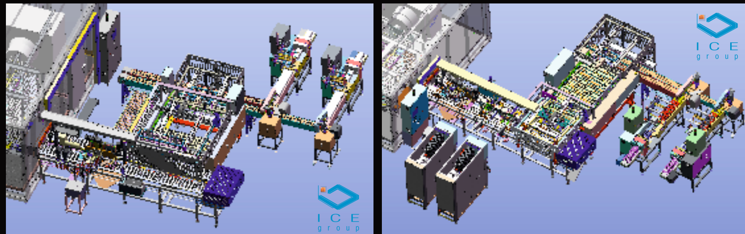
Iglo Line 12 000 D ▲ for wafer cups
