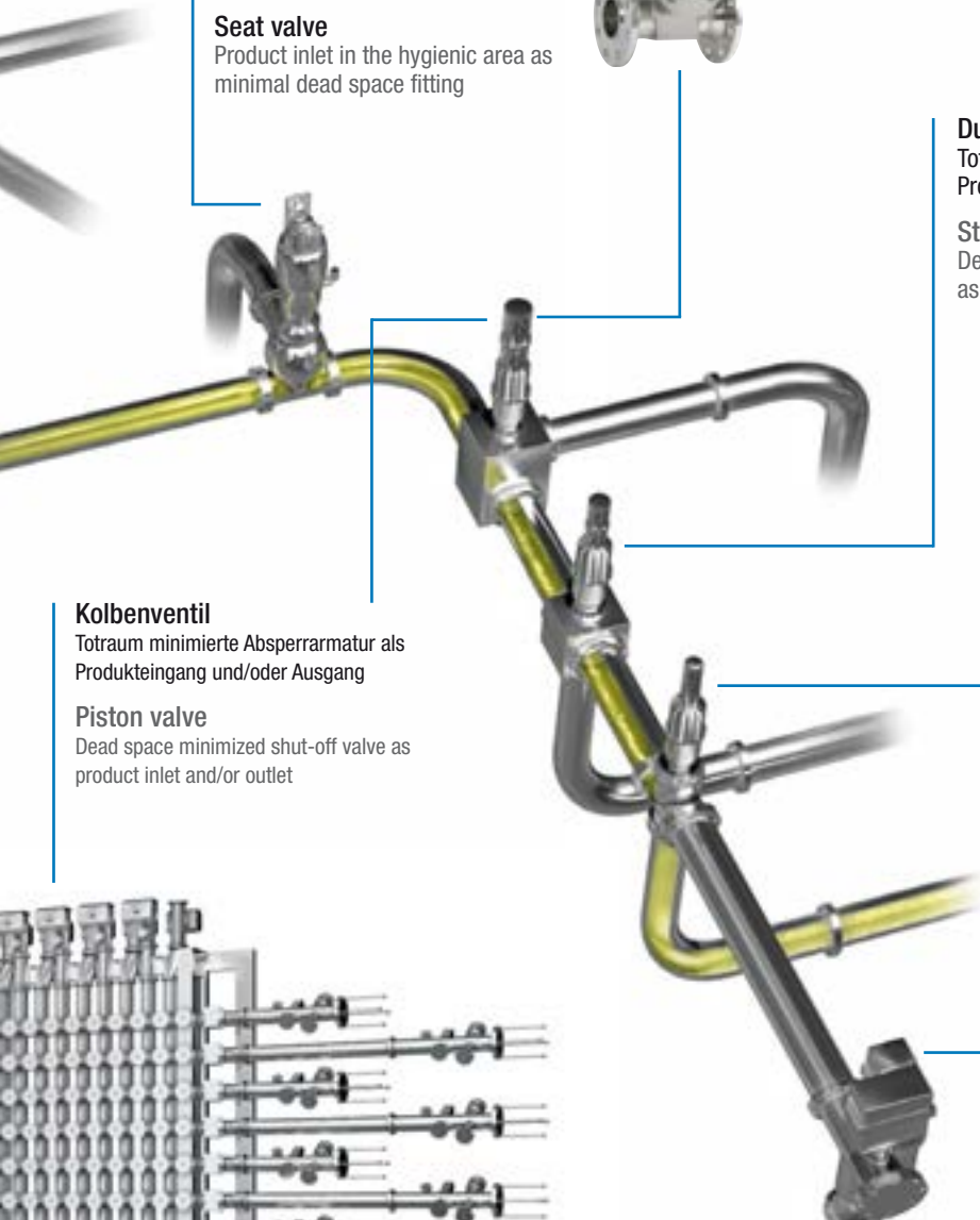
Sitzventil Produkteingang im Hygienebereich als tottraumarme Armatur
